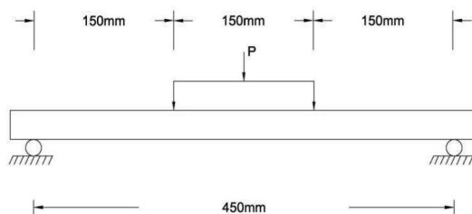
Fig 3.4.1 Test setup
